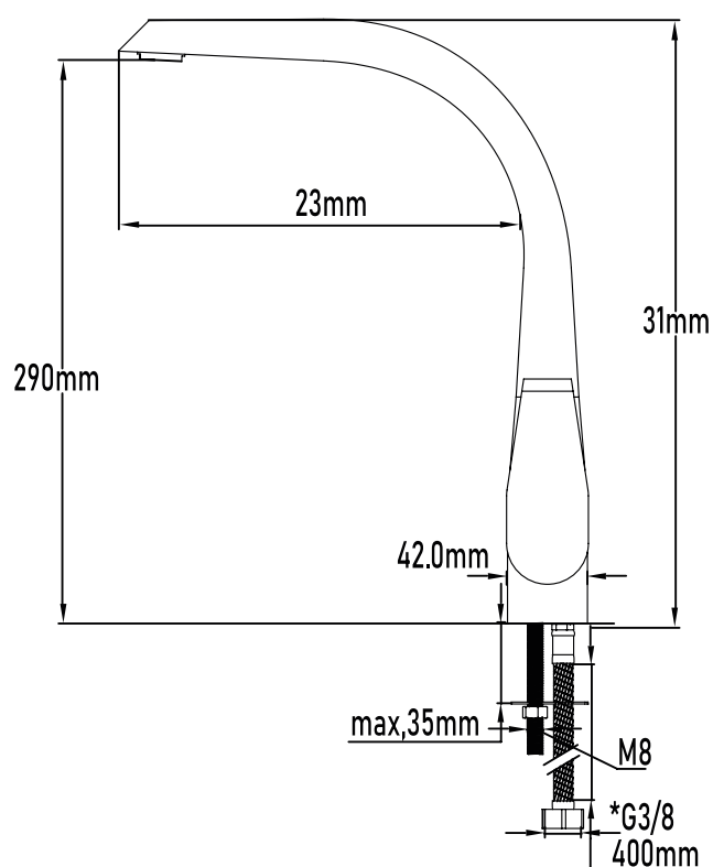
PLANO TÉCNICO
